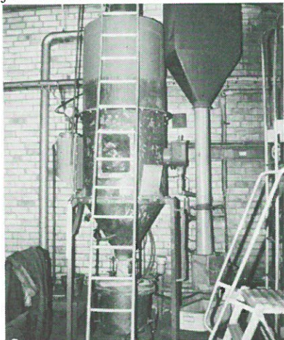
Kaskadskrubber
