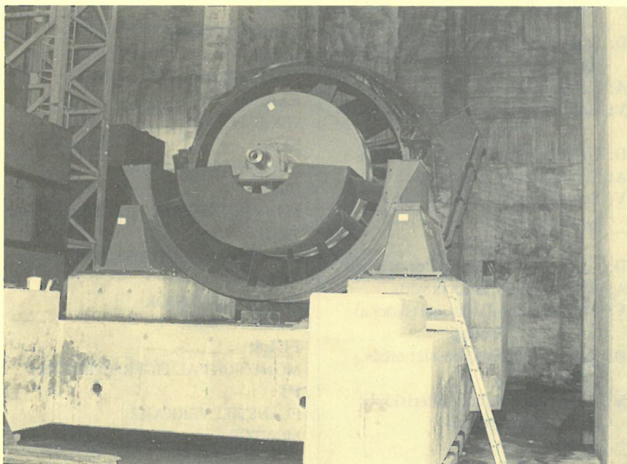
På de stora betongfundamenten ser vi PF-fläkten, delvis monterad.
