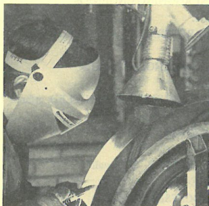
Thomas Klemmedsson svetsar vid en läge ställare med lämpligt anbringad svets- rökutsug.
