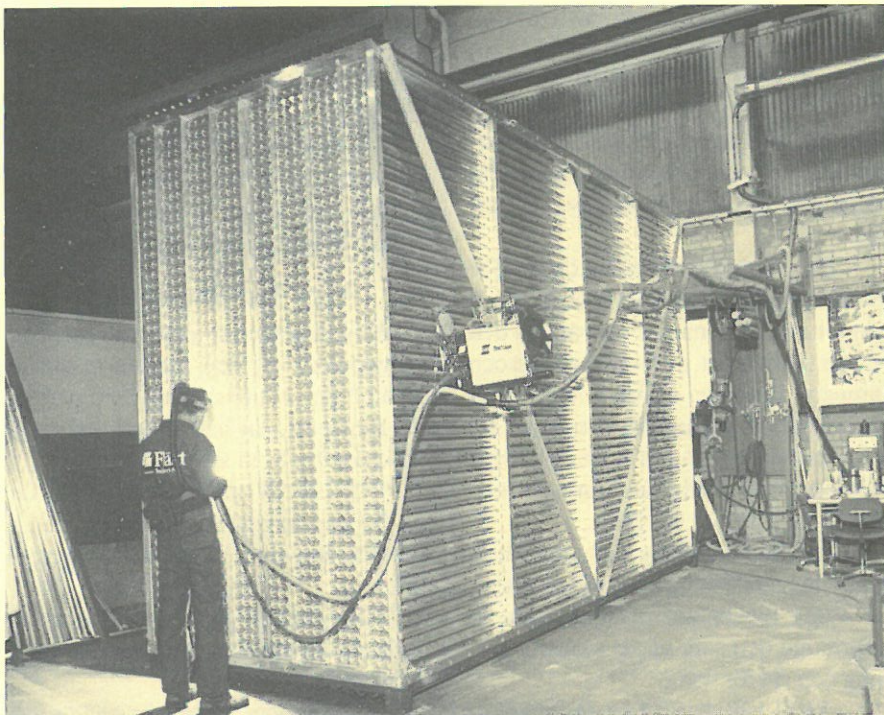
Peo Karlsson, PT56 svetsar på den jättestora värmeväxlaren.
