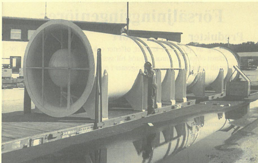
Fläkt med monterade diffussorer och ljuddämpare.
