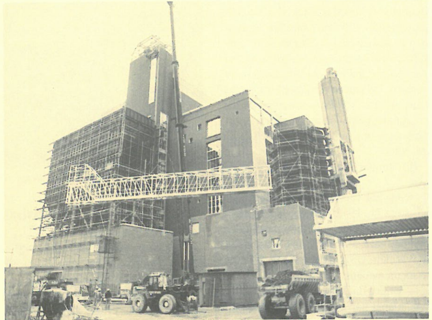
Åbyverket Örebro. Vi ser när den nästan 27 meter långa fackverkstunneln lyftas på plats. Tunneln skall monteras mellan filterkammaren (till höger i bild) och toppen på den främre silon (vänstra delen av bilden).
