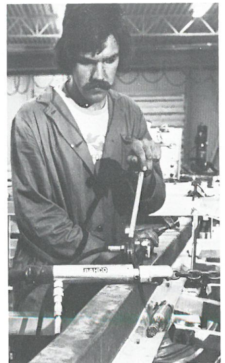
Precisionsriktning av spant före svetsning av bordläggningsplåtar med Bahco 3-tons dragcylinder.
