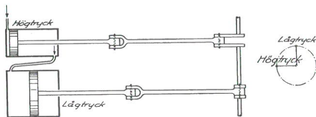
Cylinderanordning vid en compoundmaskin.
